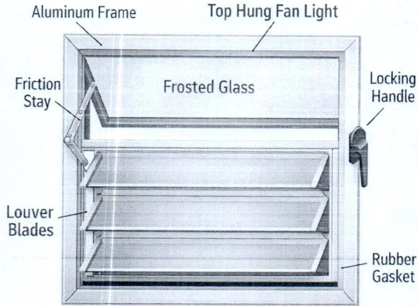
Fan Light / Ventilator 2' x 2'-6"
