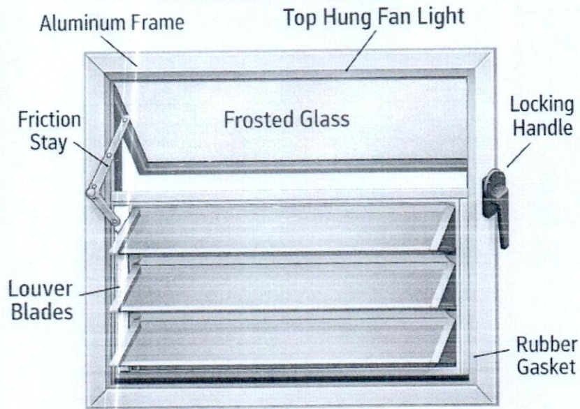
Fan Light / Ventilator 2' x 2'-6"
